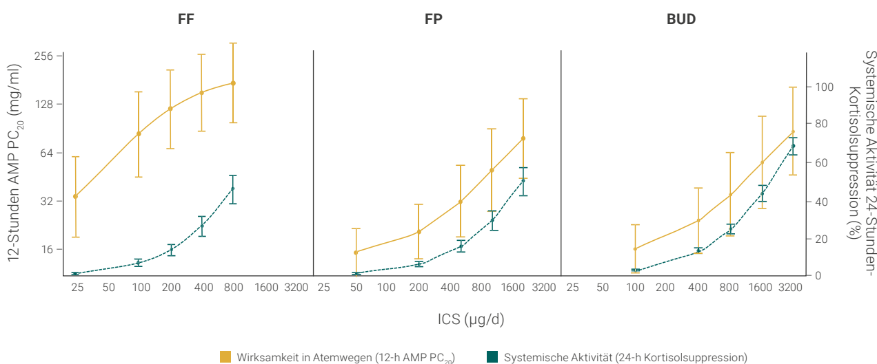
Abbildung 2: Potenz und systemische Aktivität (0 – 24 h gewichtetes Mittel der Plasmakortisol-suppression) in Abhängigkeit der ICS-Dosis bei ausgewählten Substanzen; modifiziert nach [Daley-Yates et al. 2020]. AMP PC 20 : Adenosin-Monophosphat-(AMP)-Konzentration, die das FEV 1 um ≥ 20 % reduziert; BUD: Budesonid, FEV 1 : Einsekundenkapazität, FF: Fluticasonfuroat, FP: Fluticasonpropionat, ICS: Inhalative Kortikosteroide
